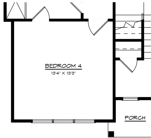
OPT. BEDROOM 4
